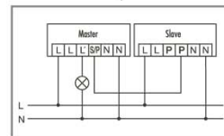
Master-Slave-Schaltung: Das Master-Gerät schaltet angeschlossene Verbraucher je nach eingestellten Parametern. Die Slave-Geräte dienen nur der Bewegungserfassung und geben bei erkannter Bewegung einen Impuls an das Master-Gerät. Achtung: Es können max. 10 Slave-Geräte an ein Master-Gerät angeschlossen werden.
